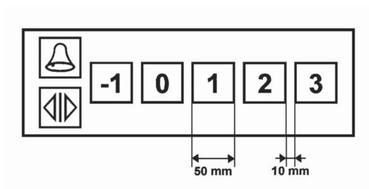
Figura G.2 – Ejemplo de disposición de una hilera de botones de presión cuadrados / Exemplo de arranjo com uma carreira de botões de pressão quadrados
